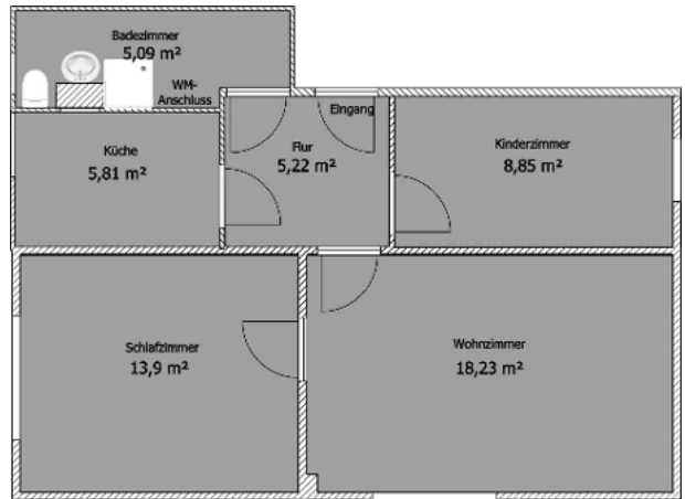
Grundriss
